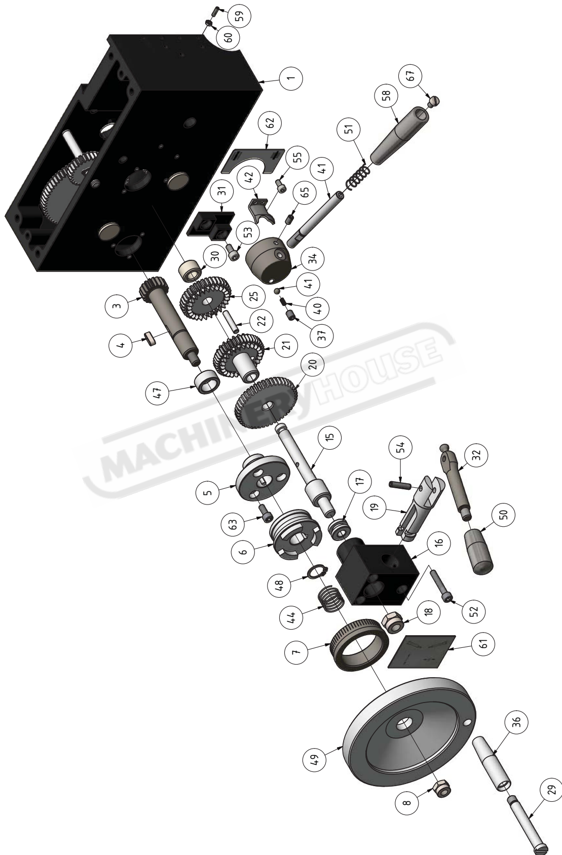
Abb.6-9: Schlosskasten - Apron
